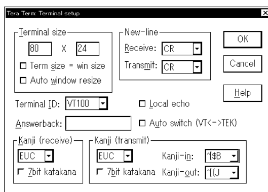
図 11.4 Tera Term Pro 設定画面
