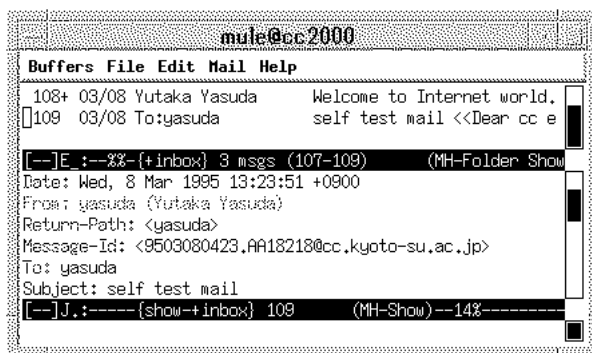
図 5.15 メールの内容の表示
