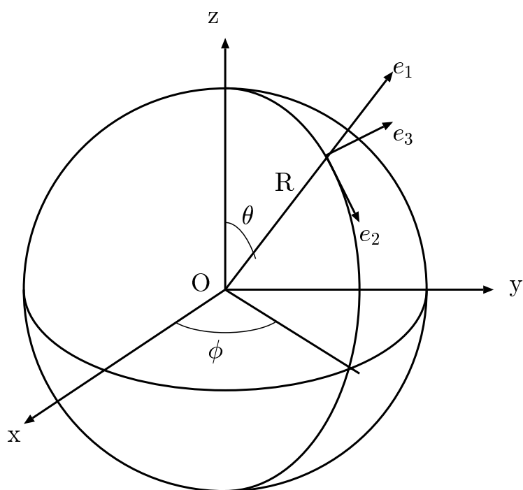
図 9.6 球面座標の直交基底
