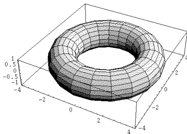
図 9.5 トーラス曲線
